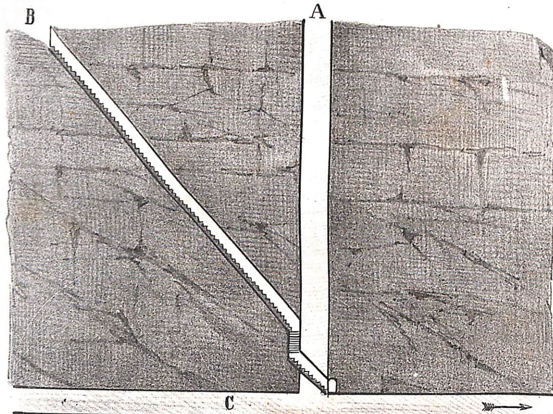
(Sezione verticale di un pozzo e di un cunicolo nell'Emissario di Claudio) (A pozzo quadrato — B cunicolo scalare — C Emissario)
